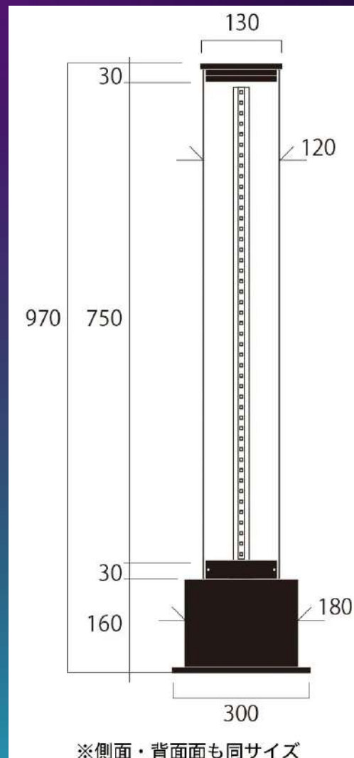
寸法
